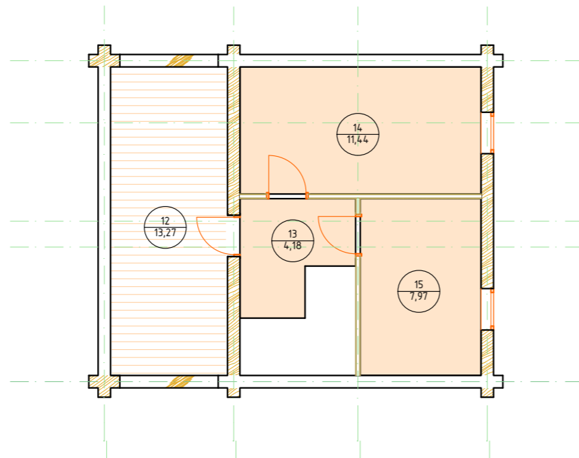
План 2-о этажа
