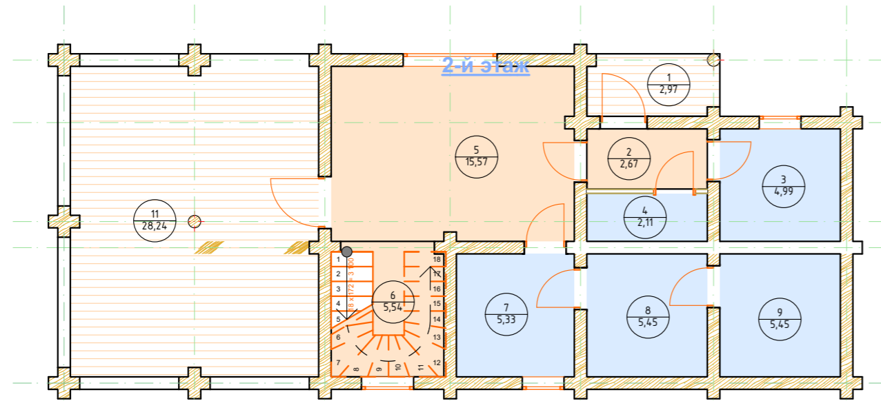
План 1-о этажа
